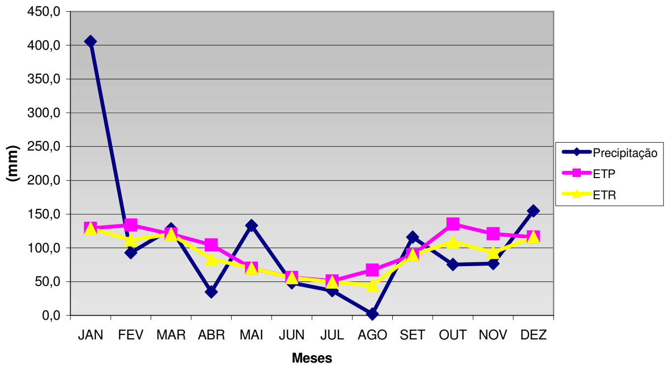
BALANÇO HÍDRICO THORNSWAITE MAITER (1955) - CAD 125 mm
